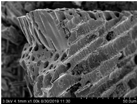
图3 曝氧竹柳炭的 SEM 图谱( \times 1000 )
