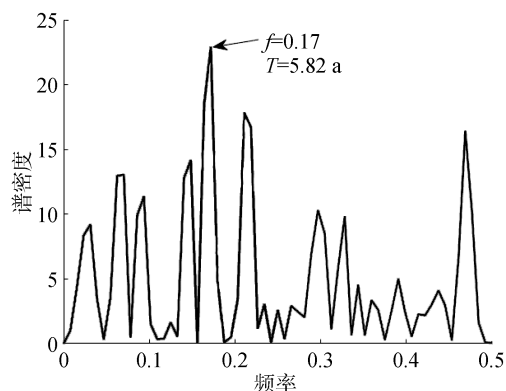
图4 登陆频次的谱估计
