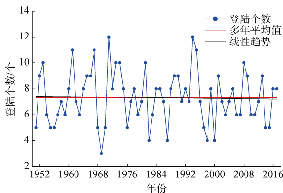
图 1 登陆中国热带气旋登陆个数的年际变化
