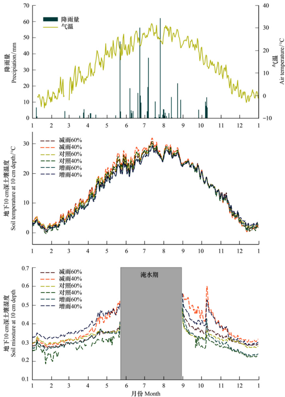
图 2 2017 年湿地气温、降雨量季节变化及不同降雨处理下地下 10 cm 深土壤温度、土壤湿度季节变化
