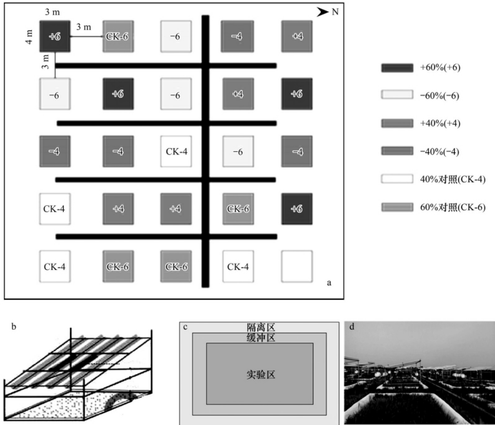
图 1 降雨控制平台实验设计图
